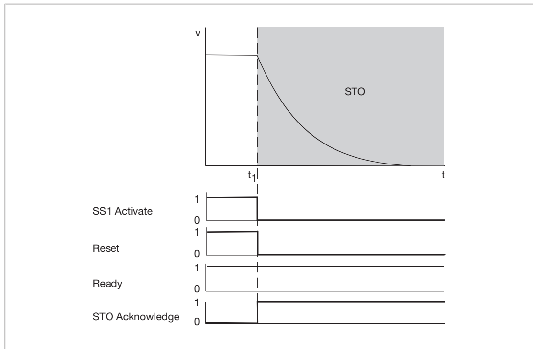
Abb.: Sicherheitsfunktion STO
