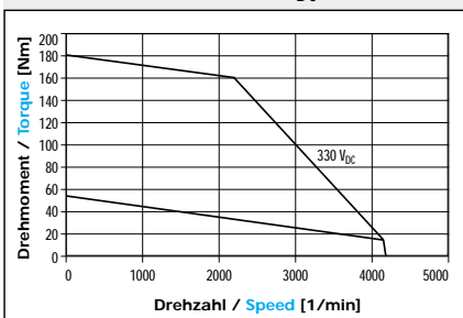
M906F 330 V DC
