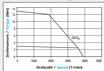
M408F 330 V DC
