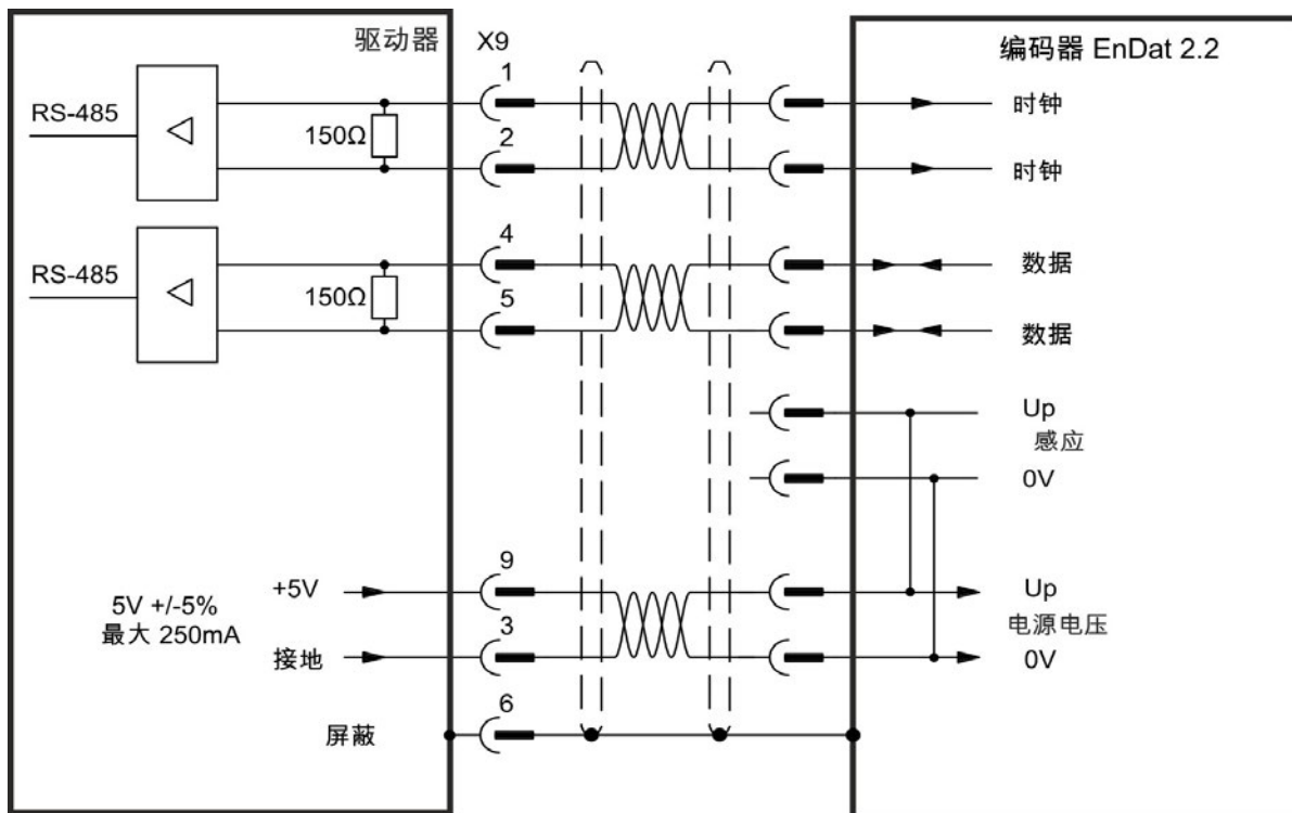
连接图
