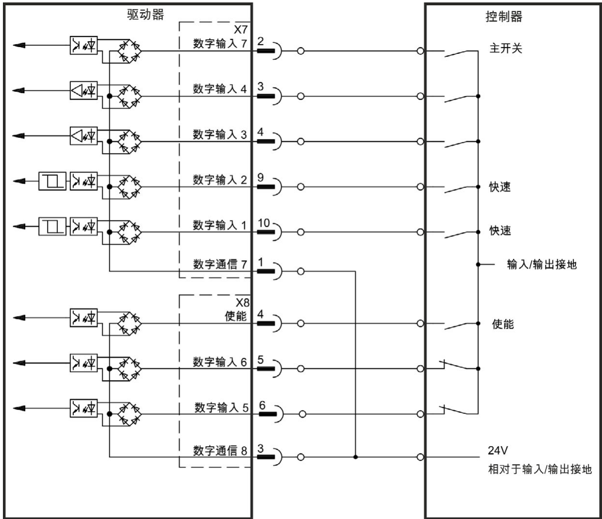
数字输入接线图(例如, 共地类型连接)
