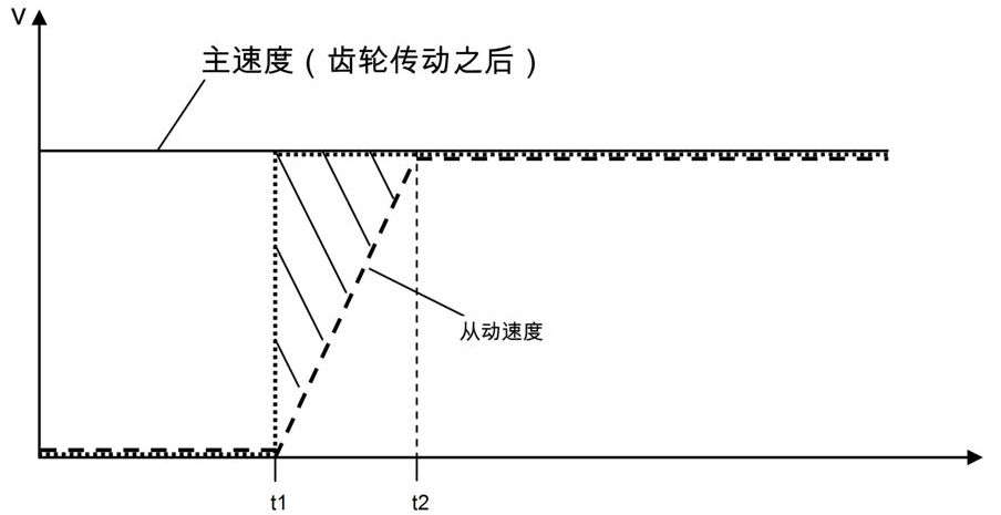
GEAR.MODE 0 加速过程
